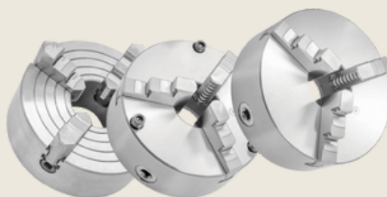
PLACAS MODELO - MONOBLOCO, REVERSÍVEIS, INDEPENDENTES.
