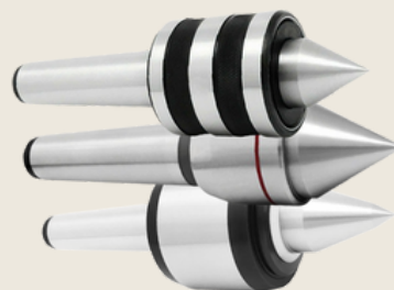
PONTOS ROTATIVOS MODELO - COMPACT, HIGH SPEED, TUBO, SUPER CARGA.
