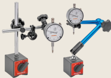
SUPOORTE MAGNÉTICO MODELO - AJUSTE FINO, ARTICULADO, FIXAÇÃO HIDRÁULICA.
