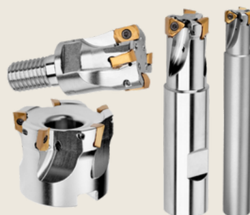
CABEÇOTES DE FRESAMENTO MODELO - CANTO A 90°.
