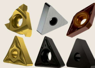
INSERTO DE TORNEAMENTO MODELO - TNMG, TCMT, TNMA, TN, TNGA, DCMT, ENTRE OUTROS MODELOS.
