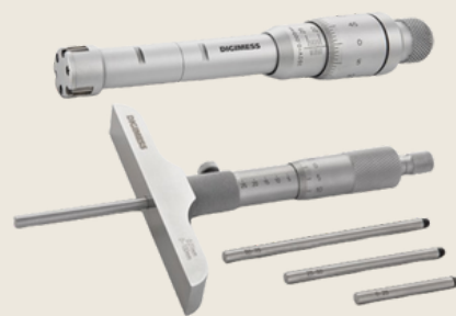
MICRÔMETRO DE PROFUNDIDADE E COM 3 PONTAS MODELO - DIGITAL, COM HASTES INTERCAMBIÁVEIS, TUBULARES.
