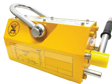
LEVANTADOR MAGNÉTICO MODELO - LS1-0.2, 0.4, 0.6, 1, 2, 3.
